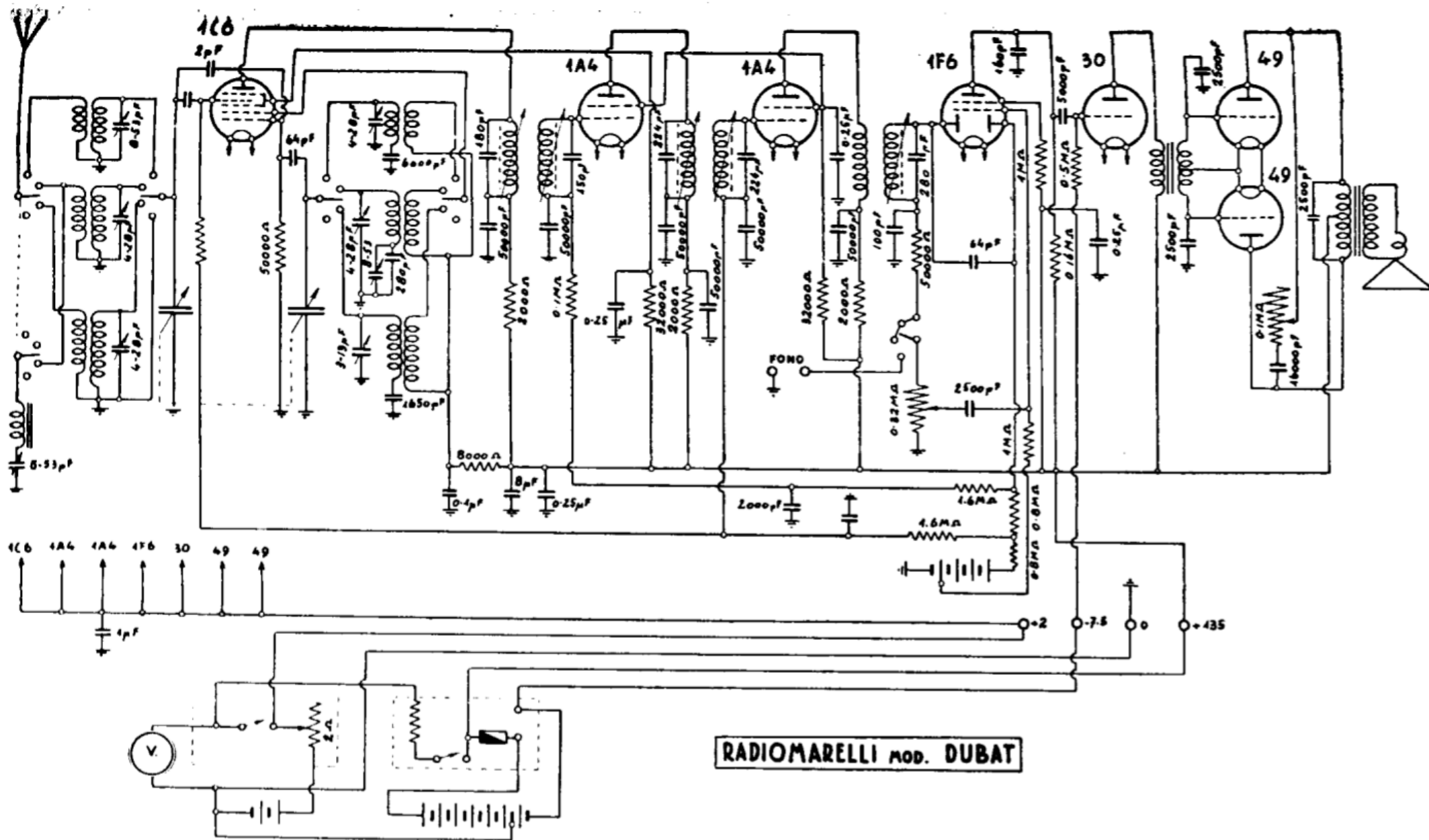
— RADIO MARELLI. — Modello « Dubat ». — Produzione 1937. — Media frequenza: 450 kHz.
